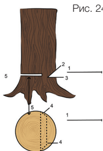
Рис. 24 Стандартный метод валки дерева (рис. 24)
